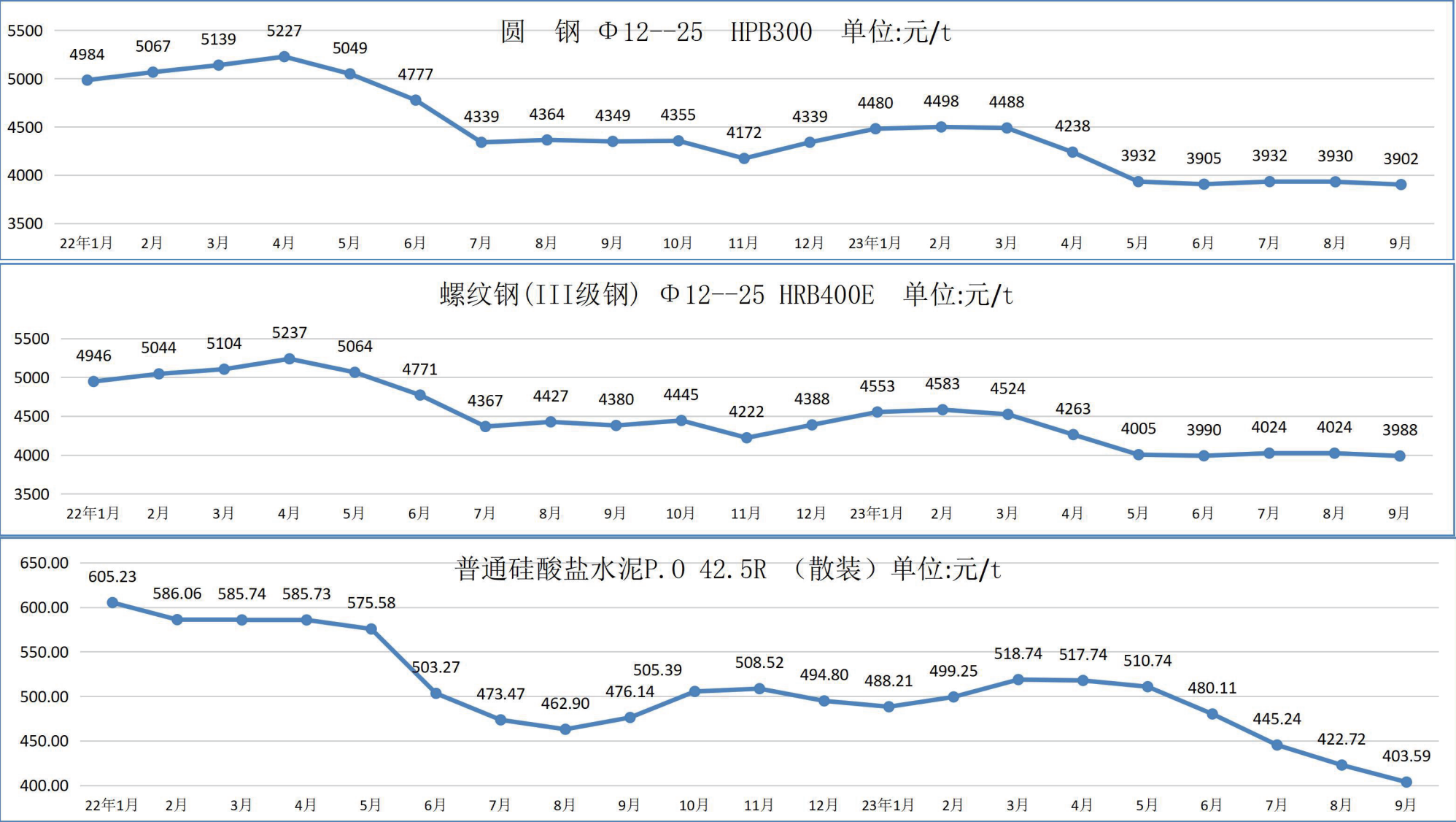
2023 年 9 月广州地区建设工程部分常用材料税前综合价格走势
