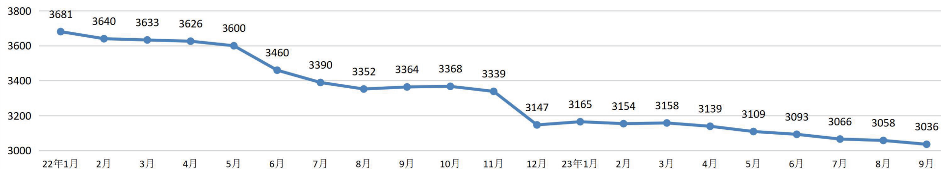
预制楼梯 钢筋含量80Kg/m 3 单位:元/m 3
