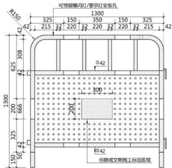
穿孔钢板铁马正立面图
