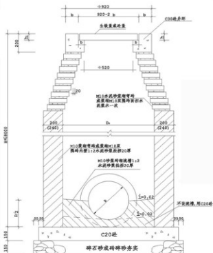
剖面图
