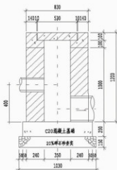
II-II 剖面图
