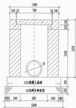
I-I 剖面图
