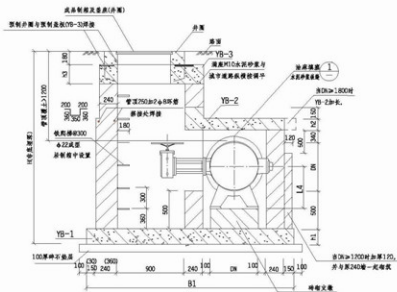
卧式蝶阀井
