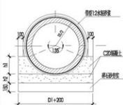
A式基础
