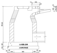
I-I 剖面图
