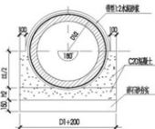
B式基础
