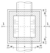
大管径检查(方井)井平面图
