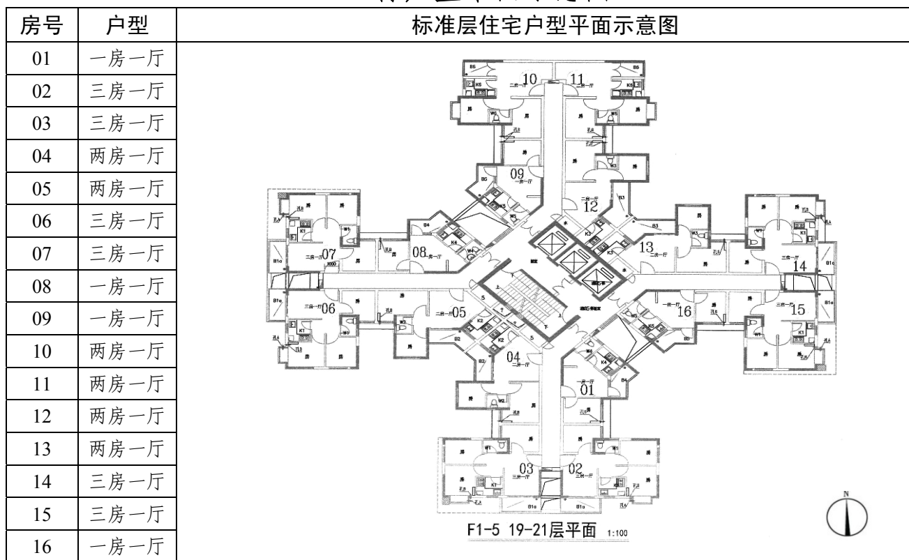
F1-5 栋户型平面示意图
